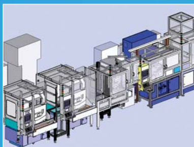
L'Allemagne commande des cellules de fabrication pour arbres de turbomoteurs
