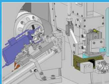
Système de mesure pour la rectification des pales d'arbre de turbomoteur
